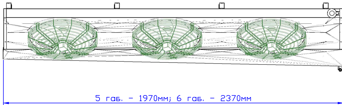
Вид спереди
