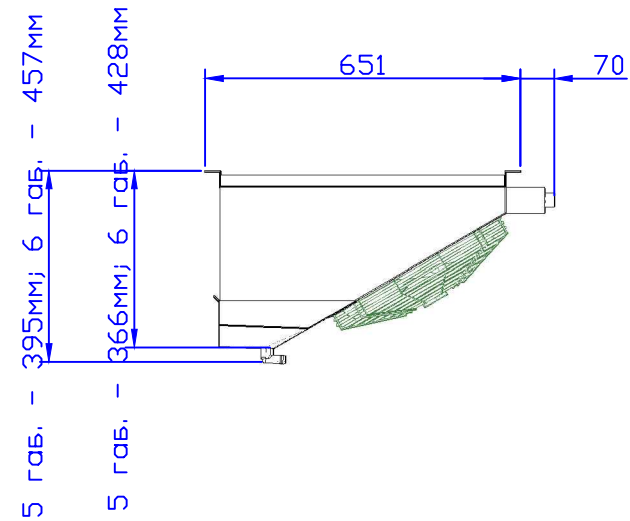
Вид слева
